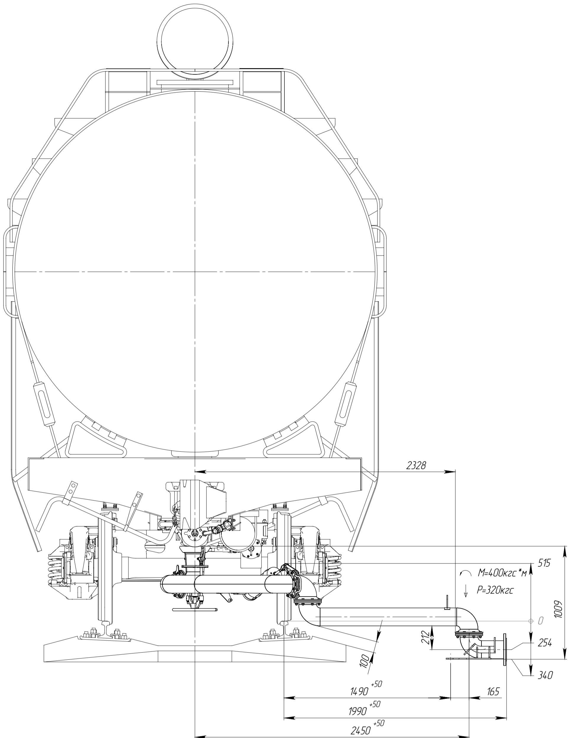
Установка нижнего слива типа УСН 6м диапазон обслуживания Монтажный чертеж
