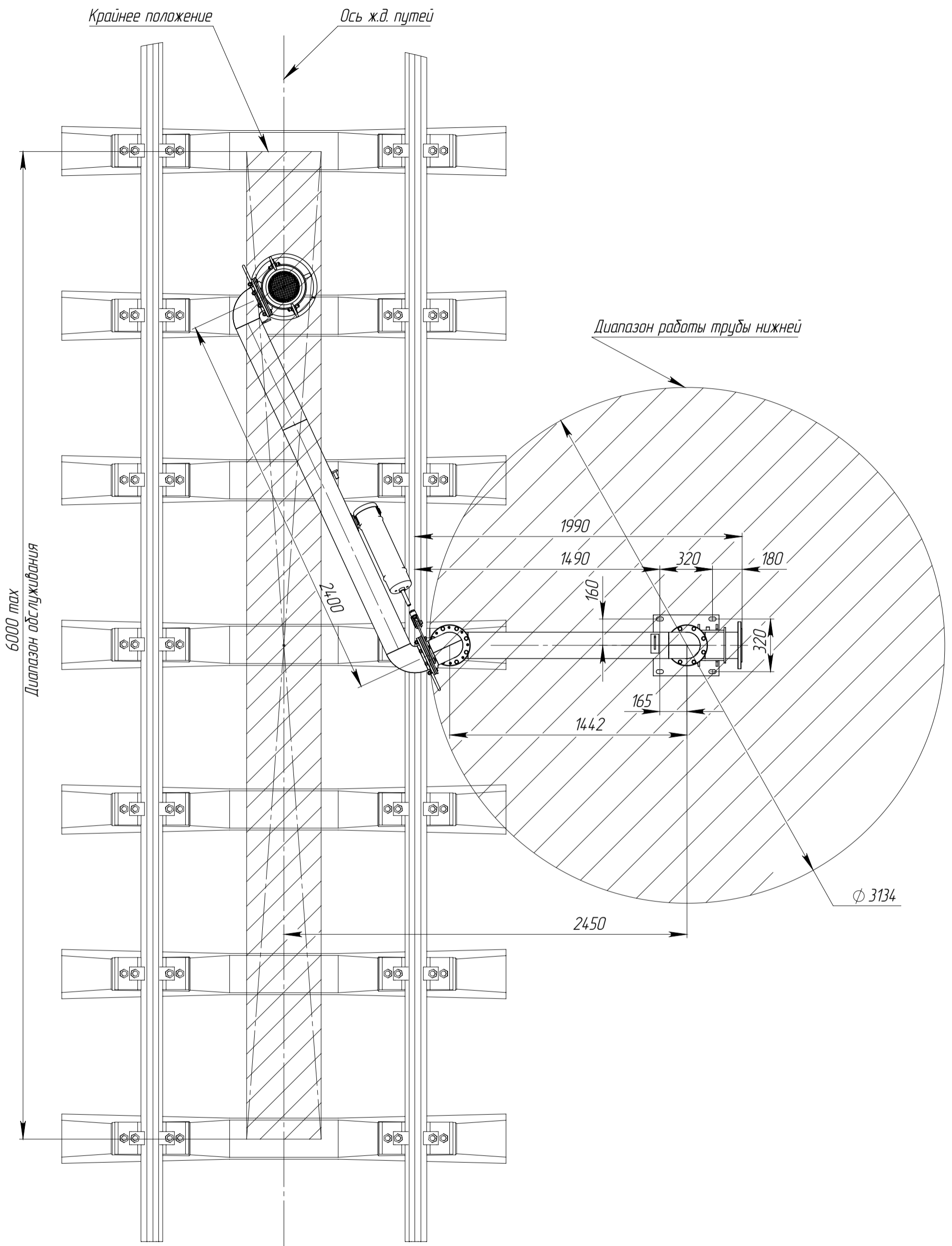
Установка нижнего слива типа УСН 6м Диаметр обслуживания
